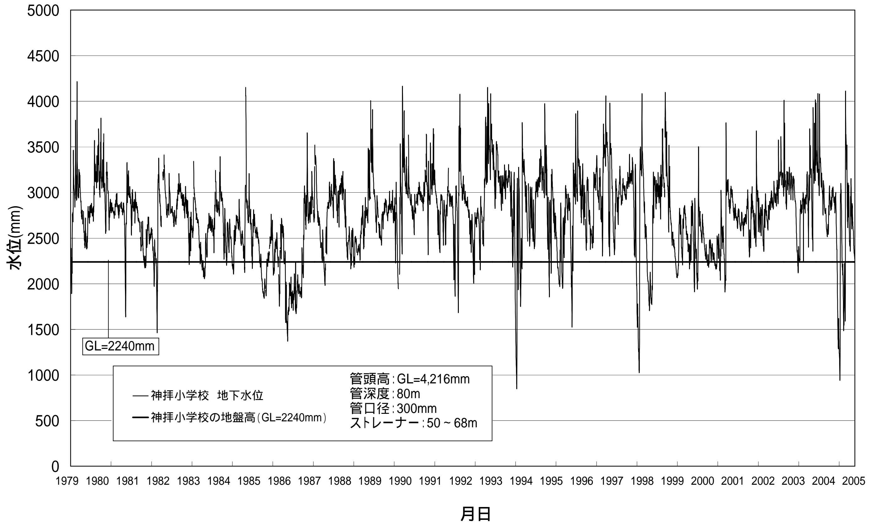
神拝小学校の地下水位 (TP基準・データ範囲: 1979年8月1日 ~ 2005年12月31日)
