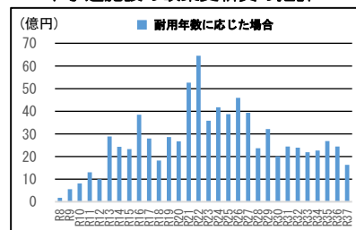
下水道施設の改築更新費の推計
