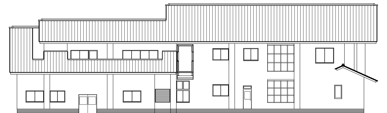
本谷温泉本館 西側立面図
