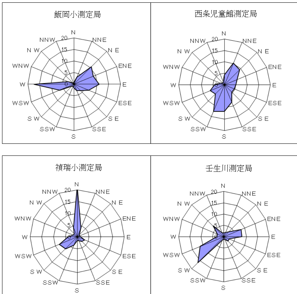
年間風配図 (単位：%)
