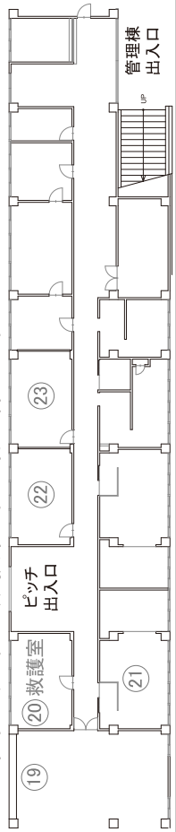
西条市ひうち陸上競技場 管理棟内諸室配置図
