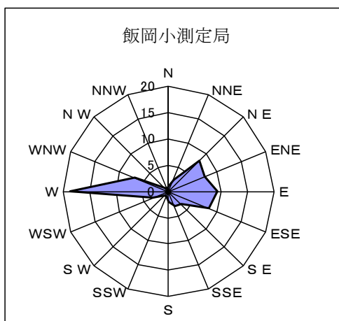
年間風配図（単位：％）
