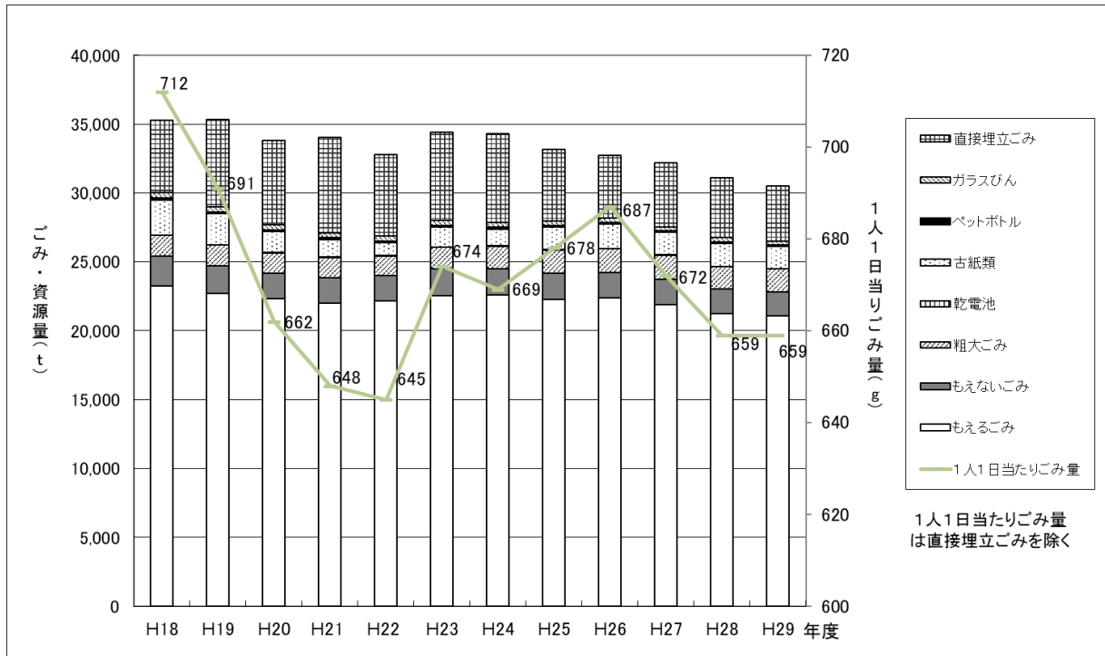
図2-2 ごみ処理量の推移（家庭系）
