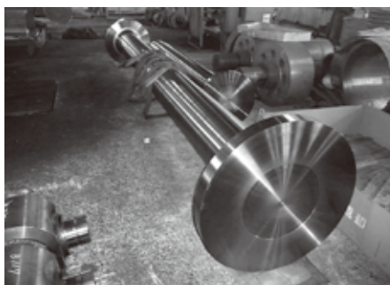
▲ 今井機械で製造した大型船舶の中間軸
