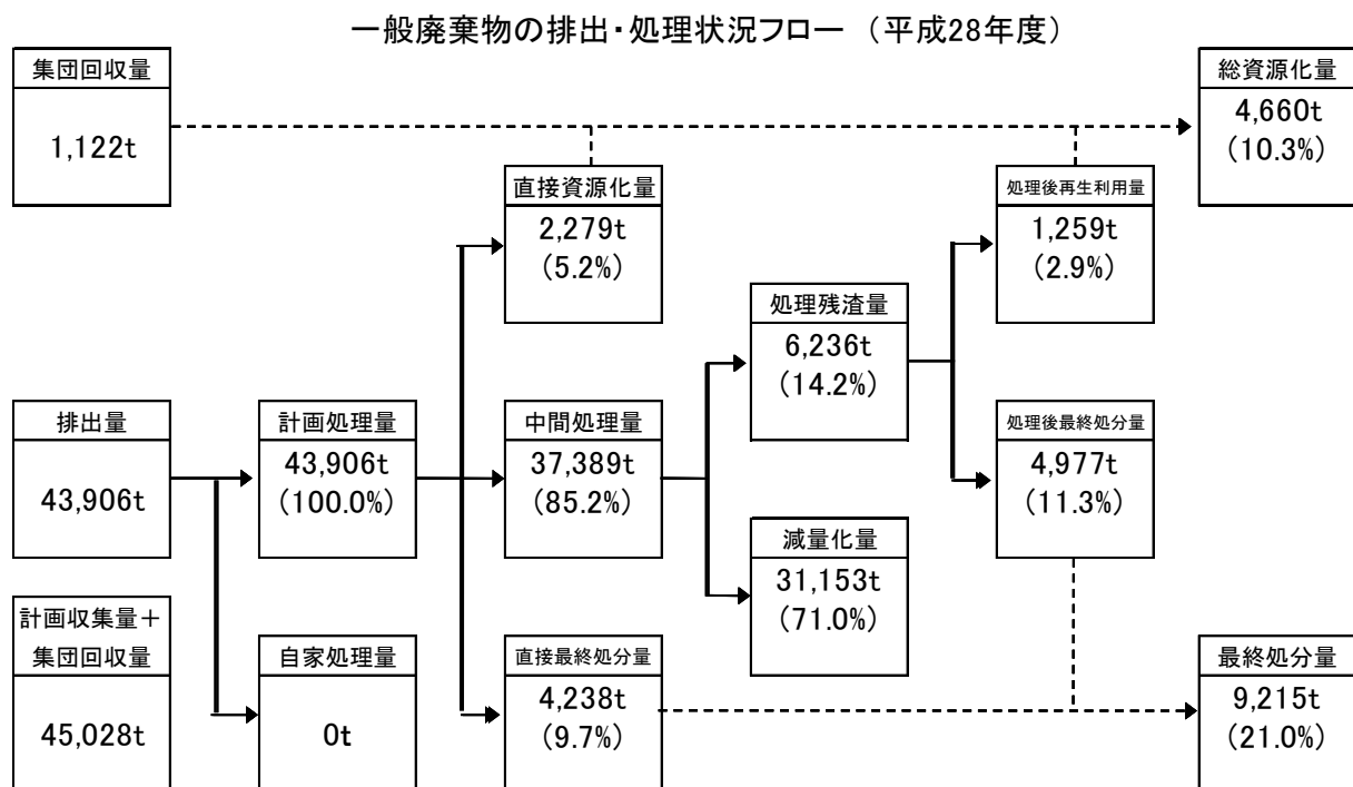
図2-1 ごみ処理フロー
