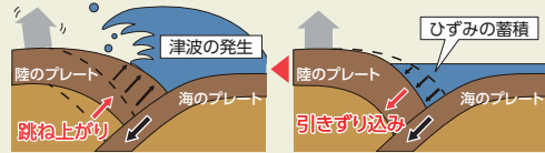
海溝型地震の仕組み
