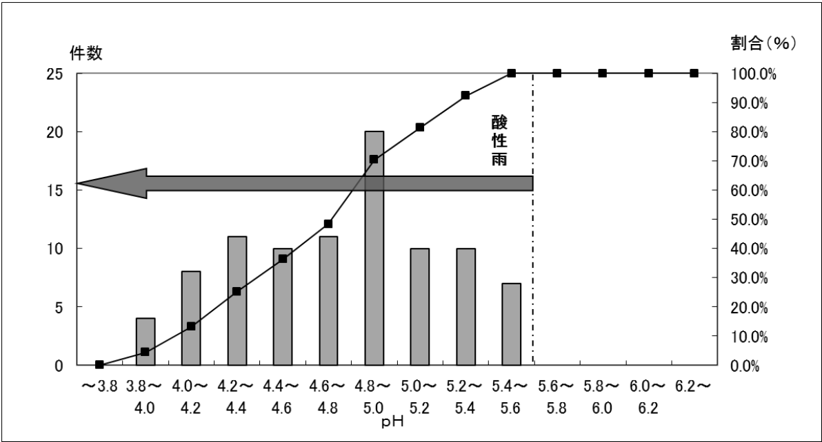
図 2-7 酸性雨濃度度数分布 (平成 26 年度)
