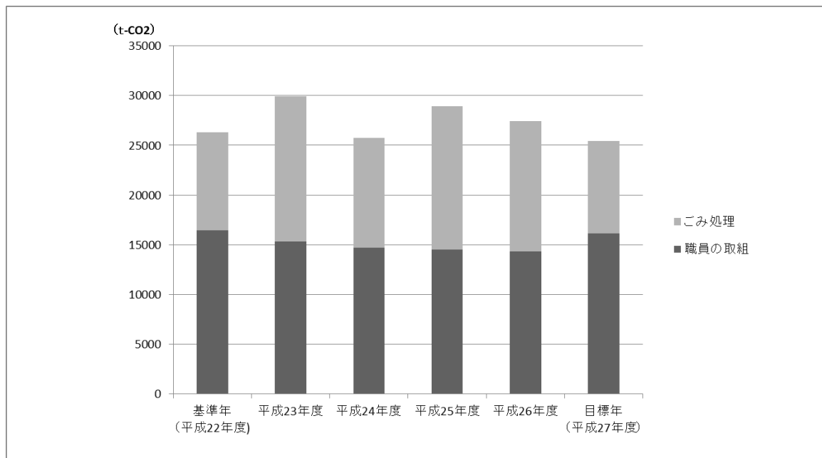
図 2-5 削減対象施設における温室効果ガス排出量の推移
