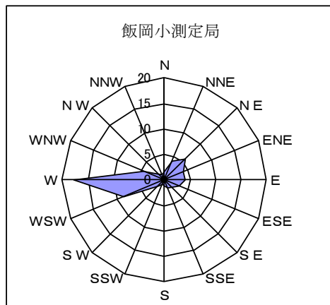
年間風配図（単位：％）
