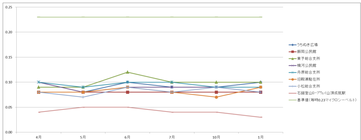
平成26年 放射線量変動状況
