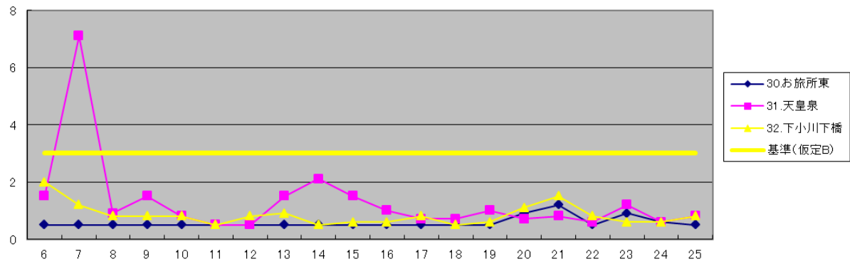
馬淵・サラサラ川水系BOD値(mg/ℓ)の年間平均値の経年変化
