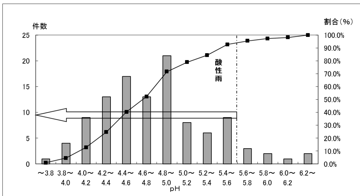
図2-7 酸性雨濃度度数分布（平成25年度）
