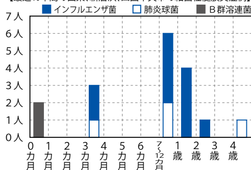
【最近10年間の西条、新居浜、四国中央市の細菌性髄膜炎症例】
