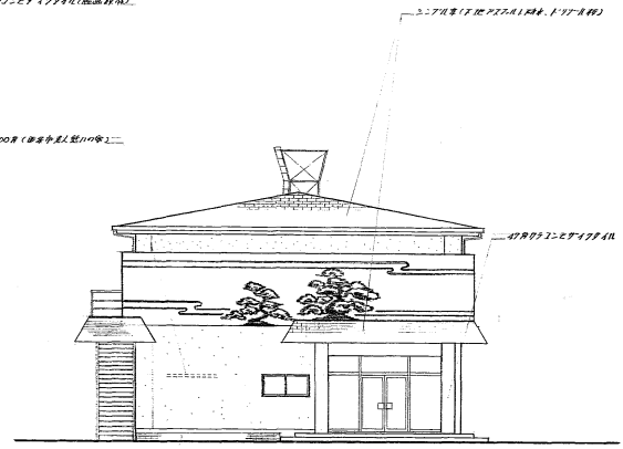
西 側立面図
