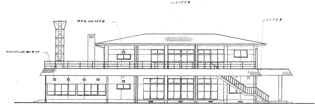
北 側立面図
