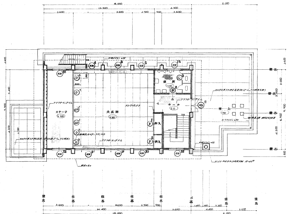
2階 平面図 1/100 △ 壁名札表示
