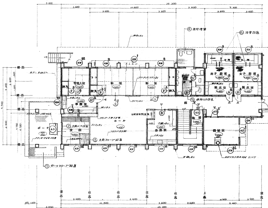
1階 平面図 1/100 (改修後) ○ G.L. 階高表示 △ 壁名札表示
