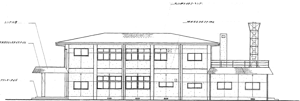
南 側立面図
