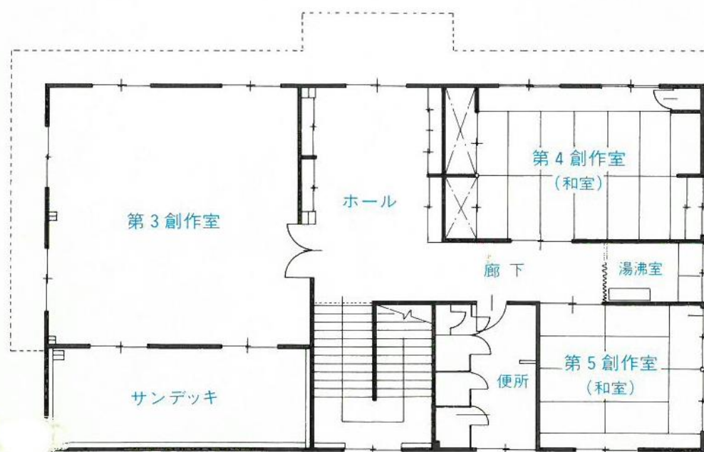
<二階平面図>
