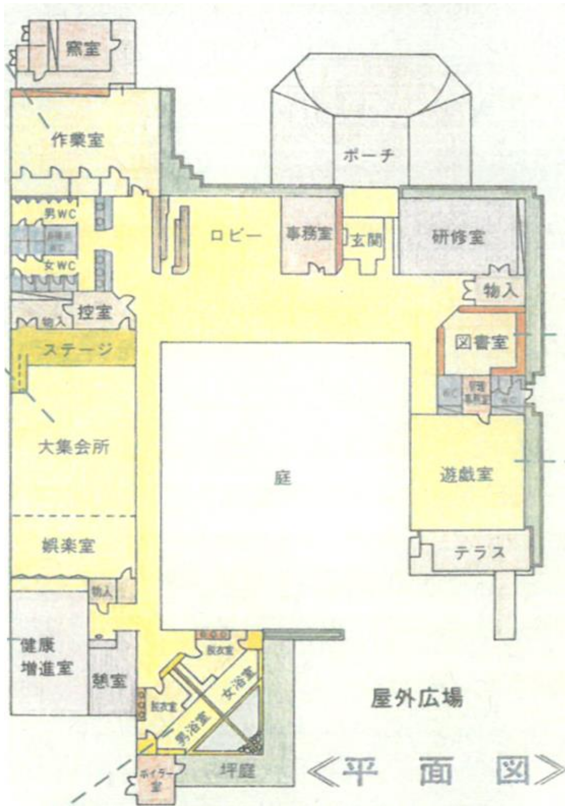
西条西部地域交流センター館内平面図
